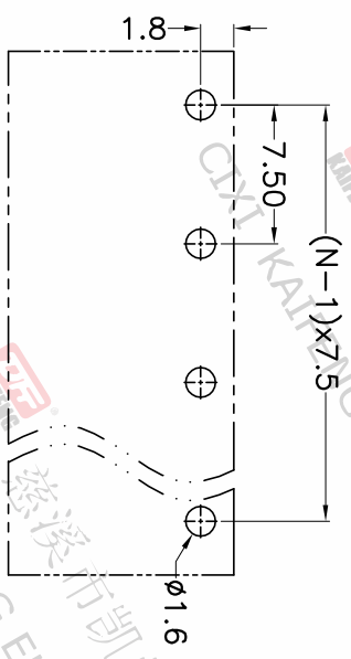
P.C.B. LAYOUT
