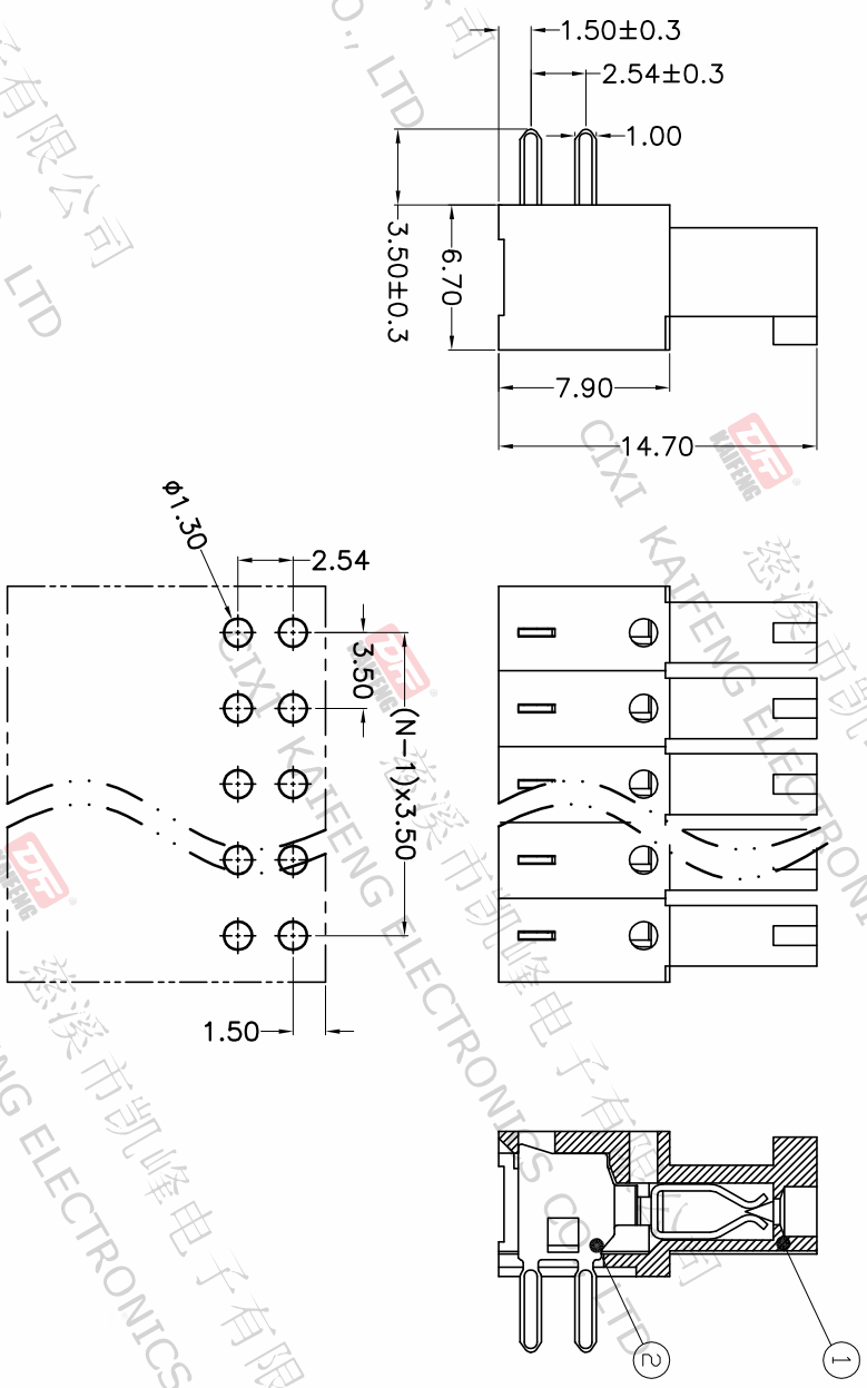
P.C.B. LAYOUT
