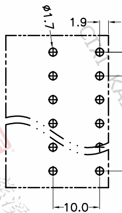
P.C.B. LAYOUT
