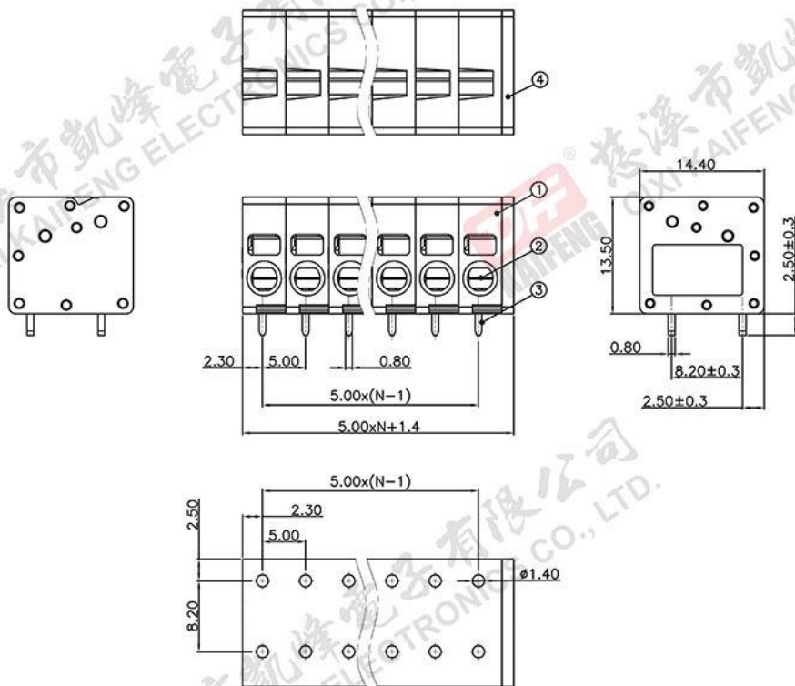
P.C.B. LAYUOT
